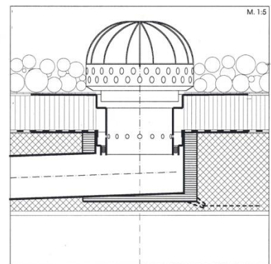
M. 1:5 Geröll Vlies Wärmedämmung Wasserdichter Belag Gefällestrich Betondecke
