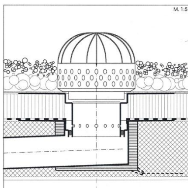
M. 1:5 Geröll / Extensivbegrünung Vlies Wärmedämmung Wasserdichter Belag Gefällestrich Betondecke
